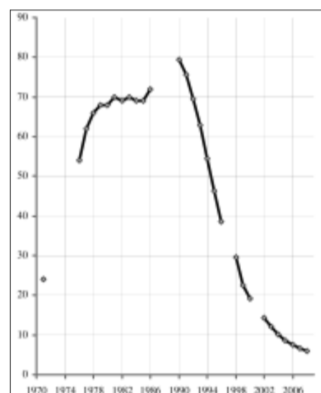
Рис. 5. Парк дождевальных и поливных машин и установок в сельскохозяйственных предприятиях России, тыс. штук
